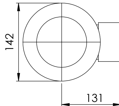
Frente do motor Motor fan cover Frente del motor (Sem escala/no scale/sin escala)
